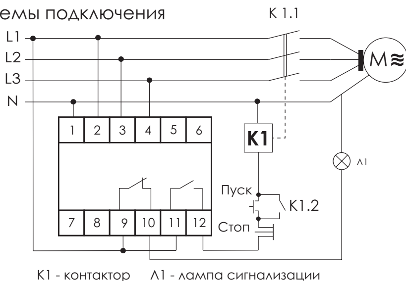
К1 - контактор Л1 - лампа сигнализации Рис.3 Схема подключения с контактором.
